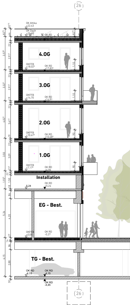
Detailschnitt
