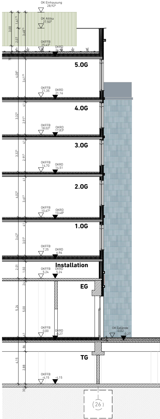
Detailschnitt
