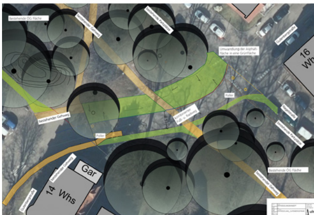
Entsiegelungskonzept - Gutenbergstraße
